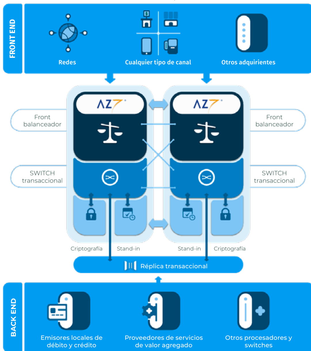
Esquema básico de Activo-Activo de AZ7®.
